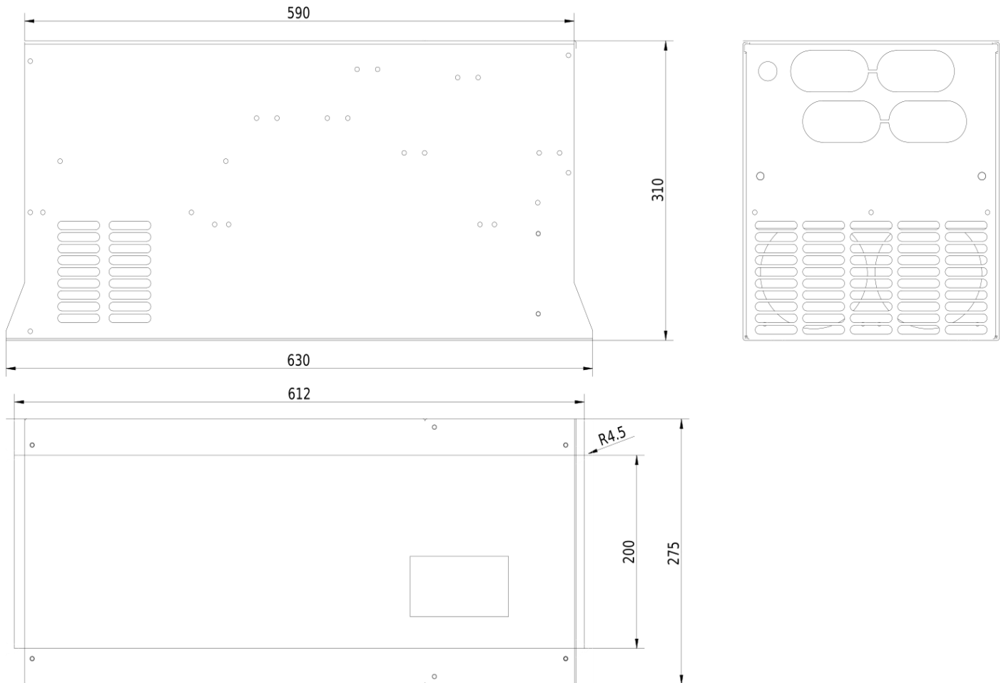
Rozmerový výkres V900 - 90kW 4T0900
