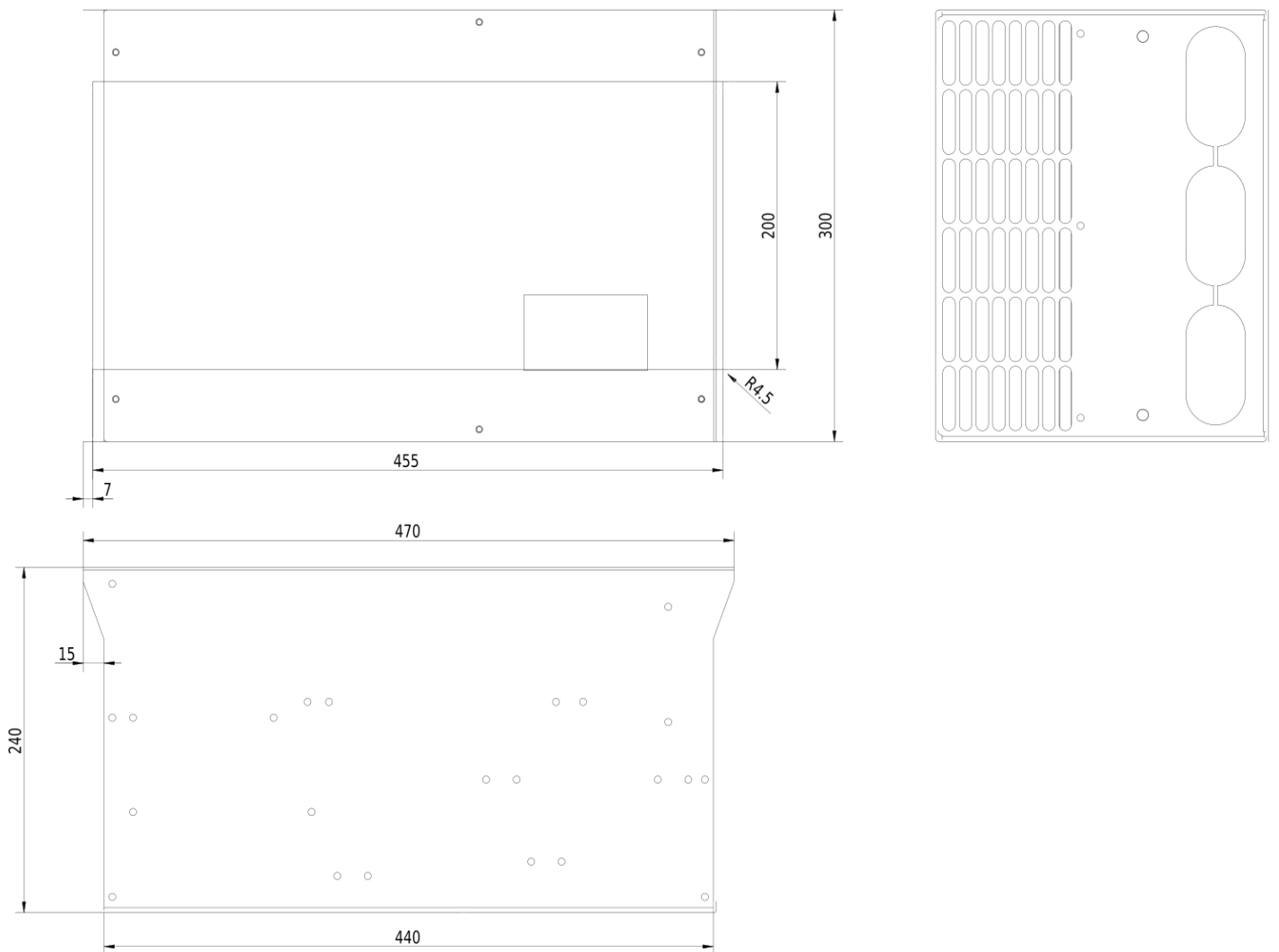
Rozmerový výkres V900 - 75kW 4T0750
