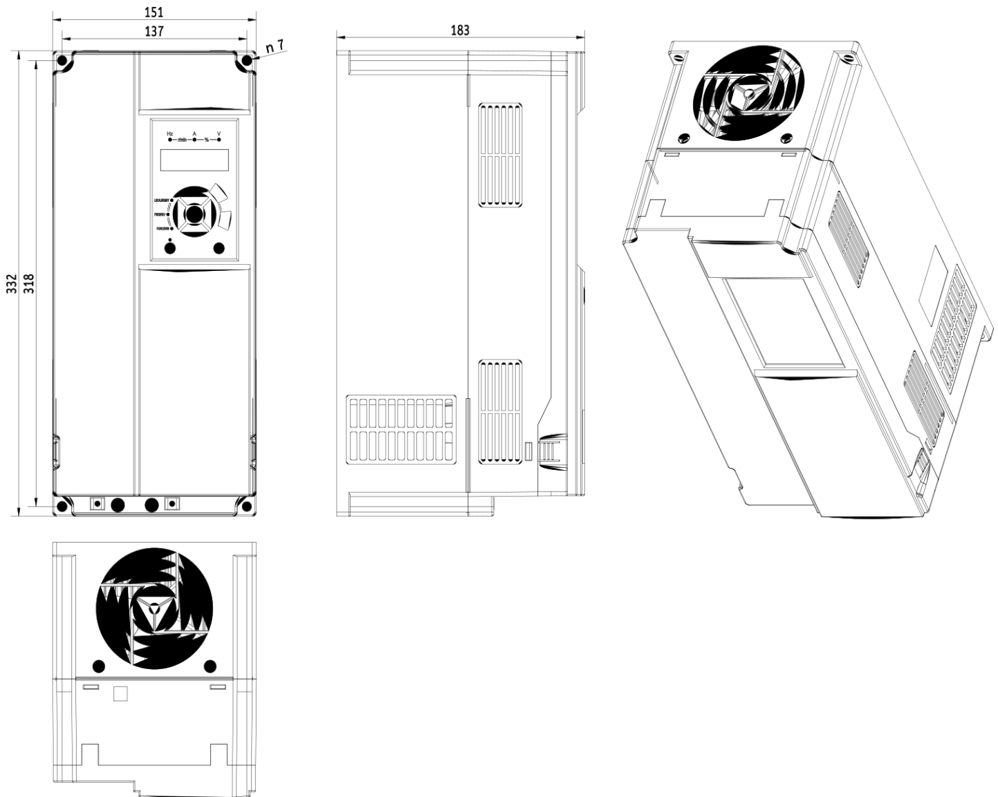
Rozmerový výkres V900 - 30kW 4T0300
