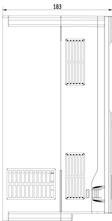
Rozmerový výkres V900 - 18,5kW 4T0185
