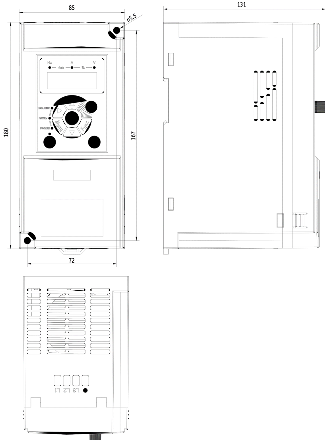
Rozmerový výkres V900 - 7,5kW 4T0075
