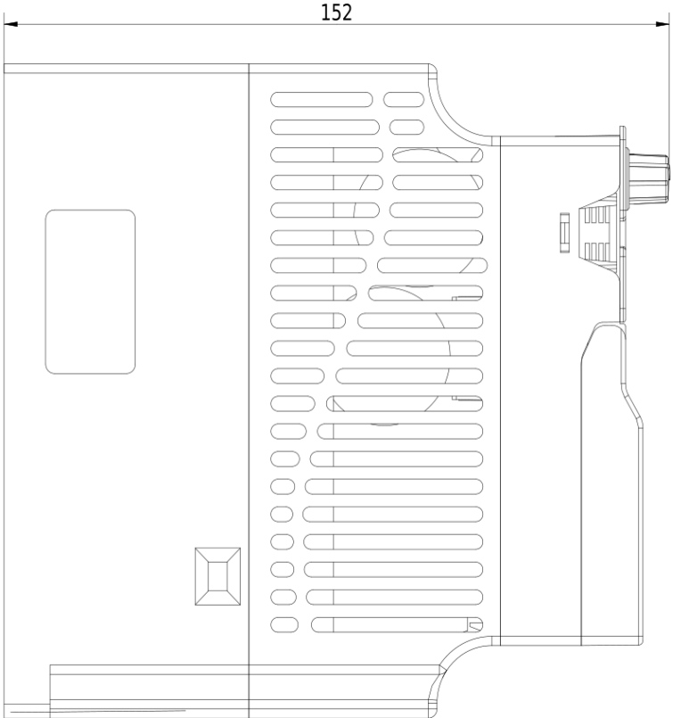
Rozmerový výkres V800 - 0,75kW 4T0007
