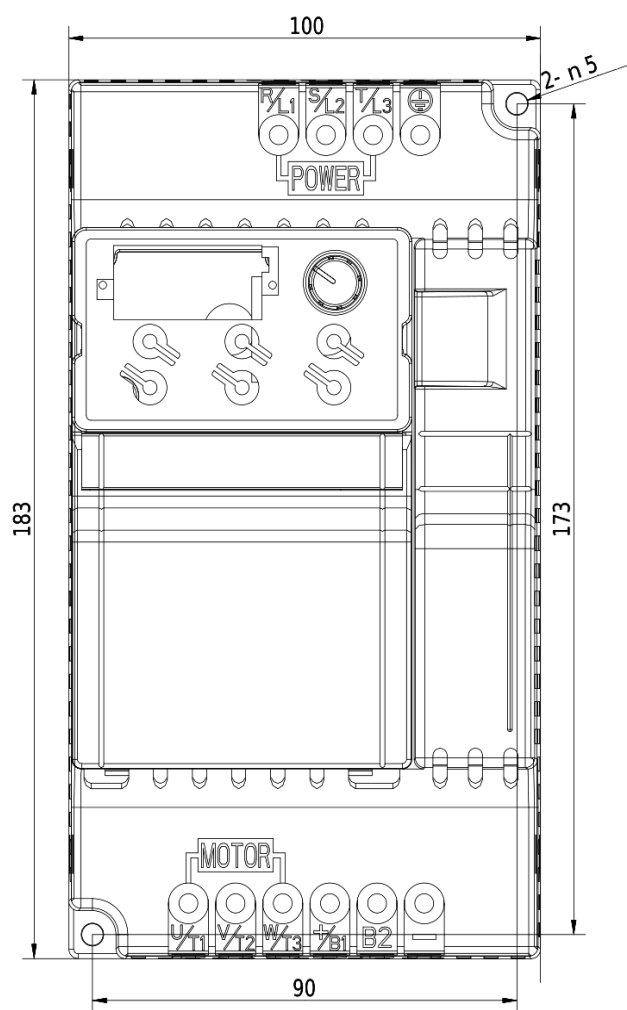
Rozmerový výkres V800 - 4,0kW 2S0040
