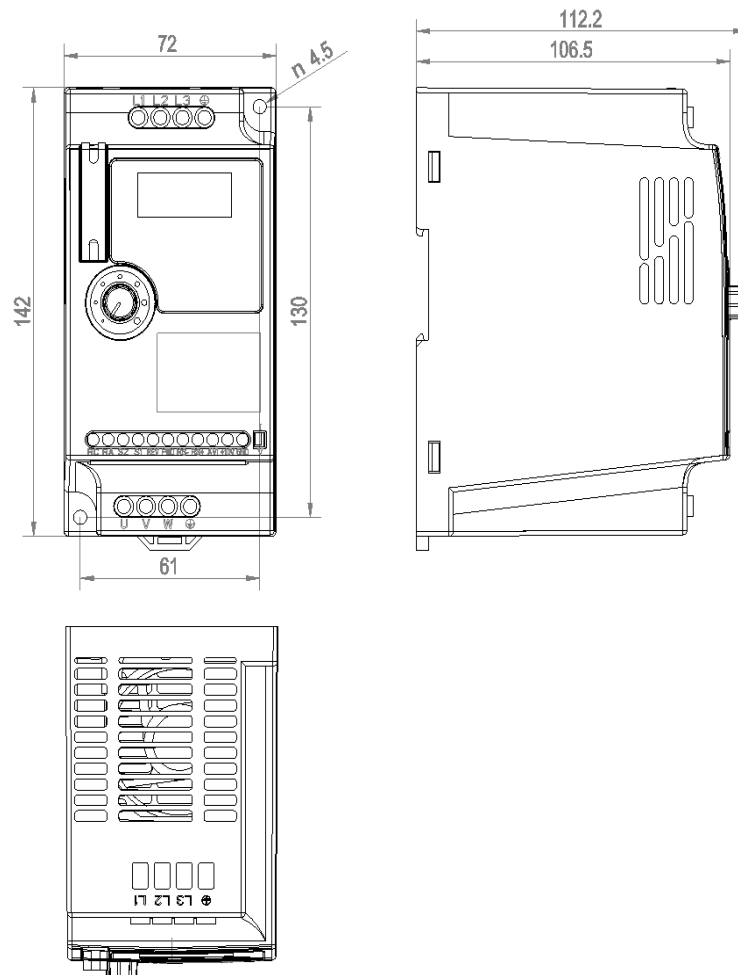
Rozmerový výkres A550 PLUS - 0,4kW 4T0004
