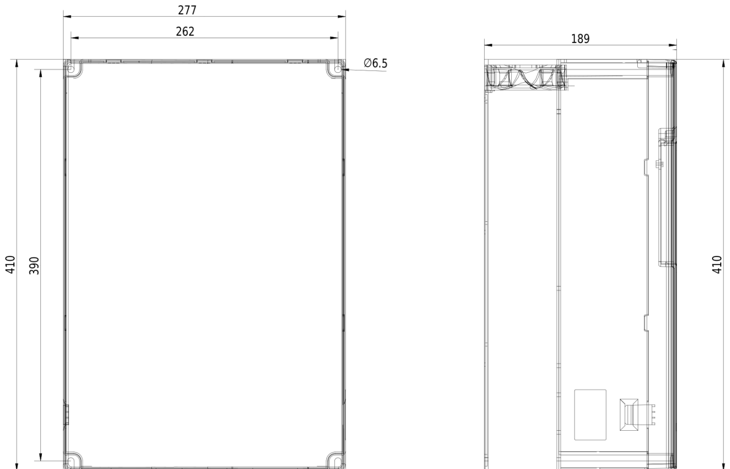
Rozmerový výkres V810 - 30kW 4T0300
