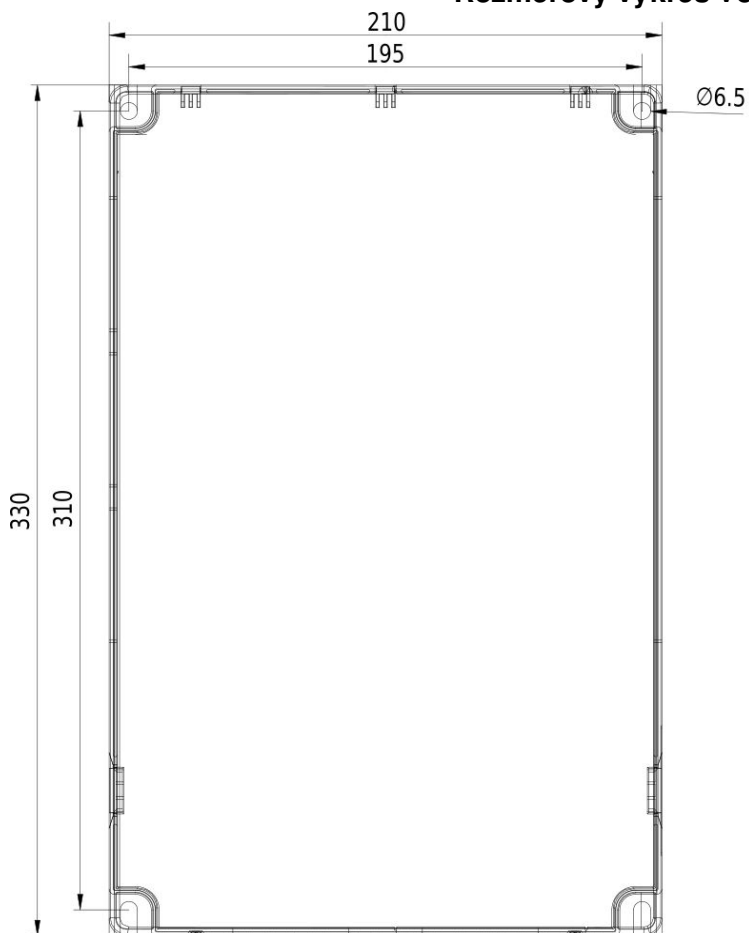
Rozmerový výkres V8 10 - 15kW 4T0 150
