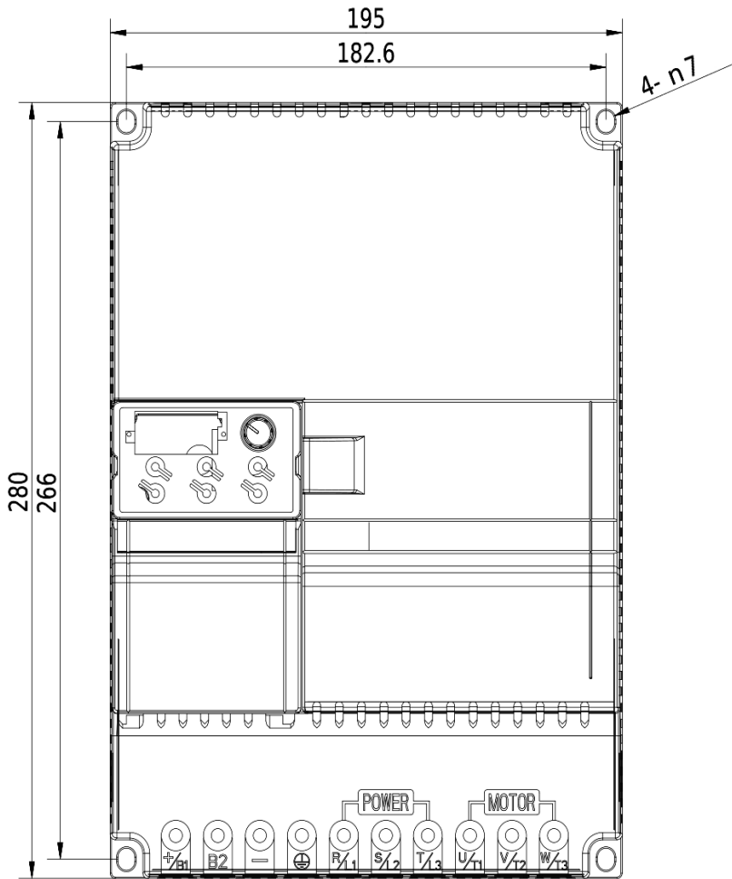
Rozmerový výkres V800 - 22kW 4T0220
