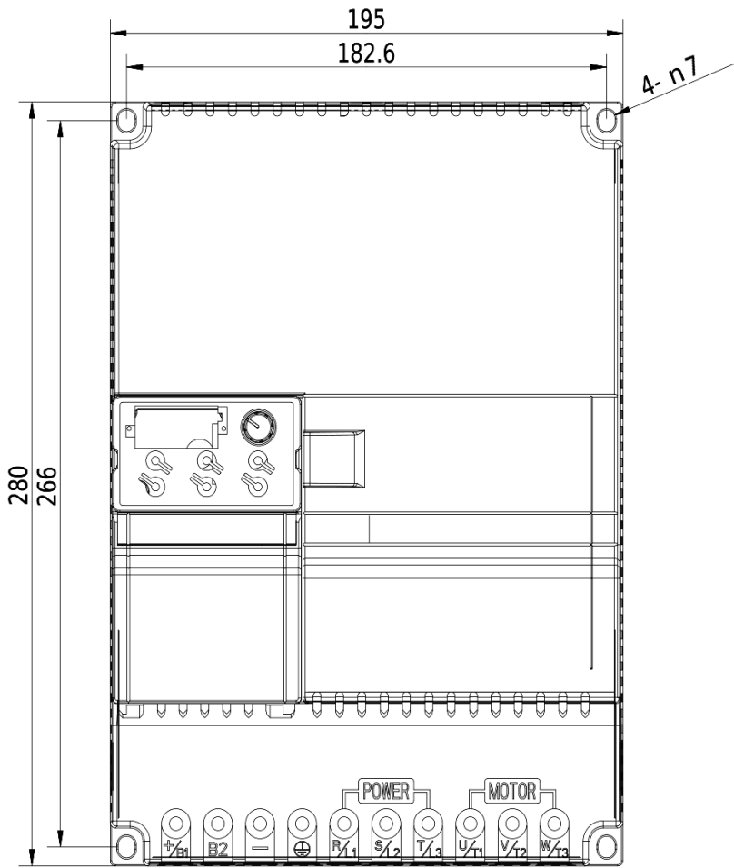
Rozmerový výkres V800 - 18,5kW 4T0185
