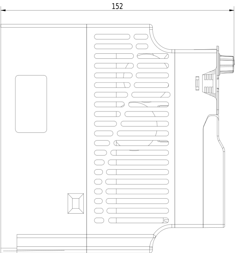
Rozmerový výkres V800 - 1,5kW 4T0015
