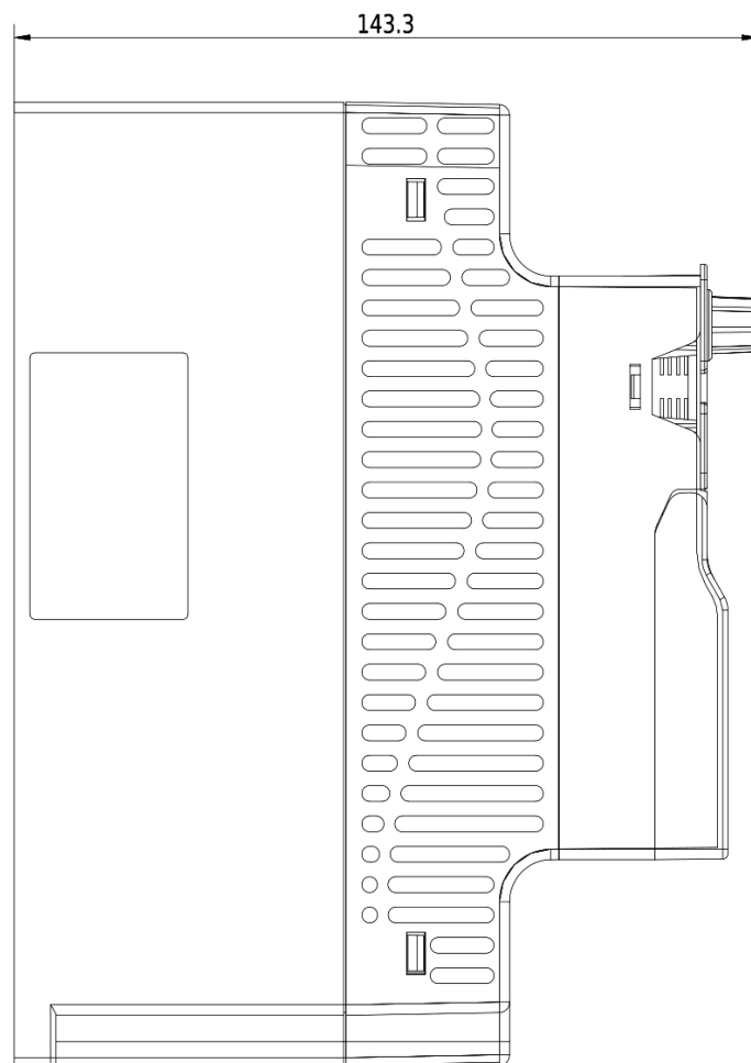
Rozmerový výkres V800 - 3,0kW 2S0030
