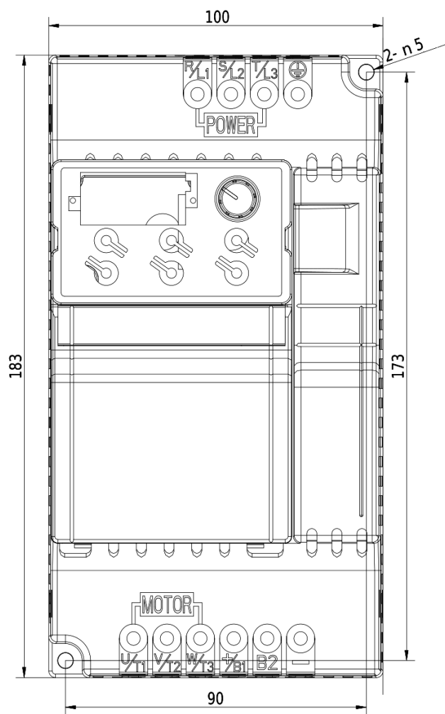
Rozmerový výkres V800 - 3,0kW 2S0030
