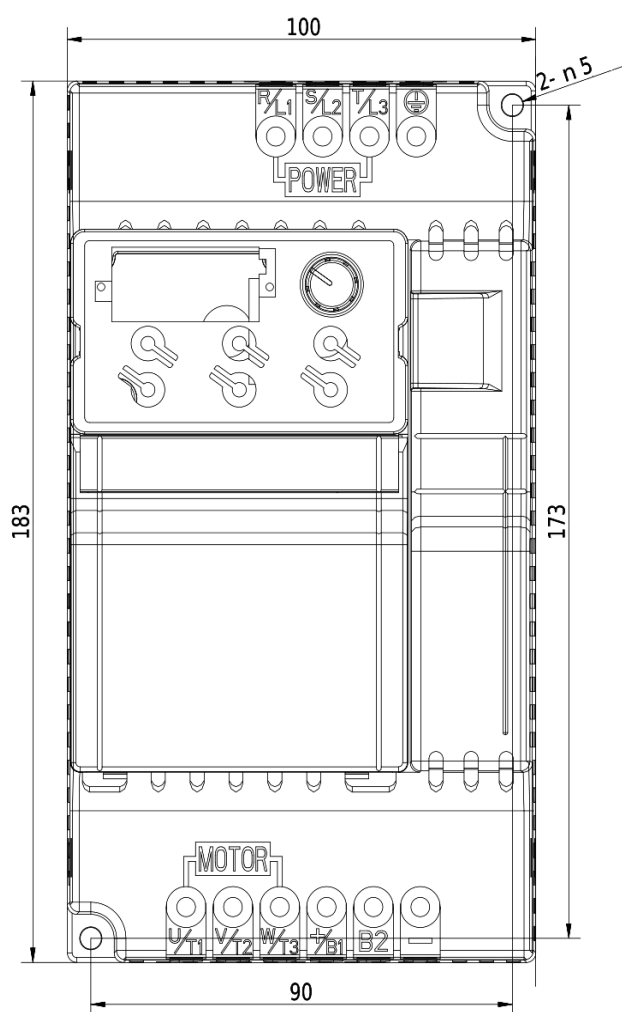
Rozmerový výkres V800 - 2,2kW 2S0022
