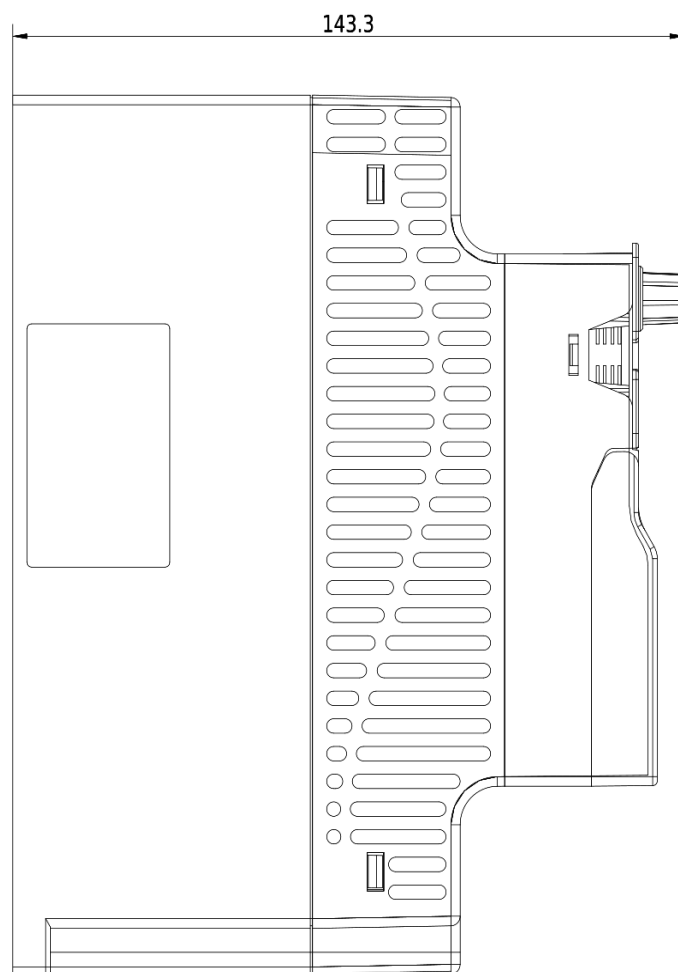
Rozmerový výkres V800 - 2,2kW 2S0022
