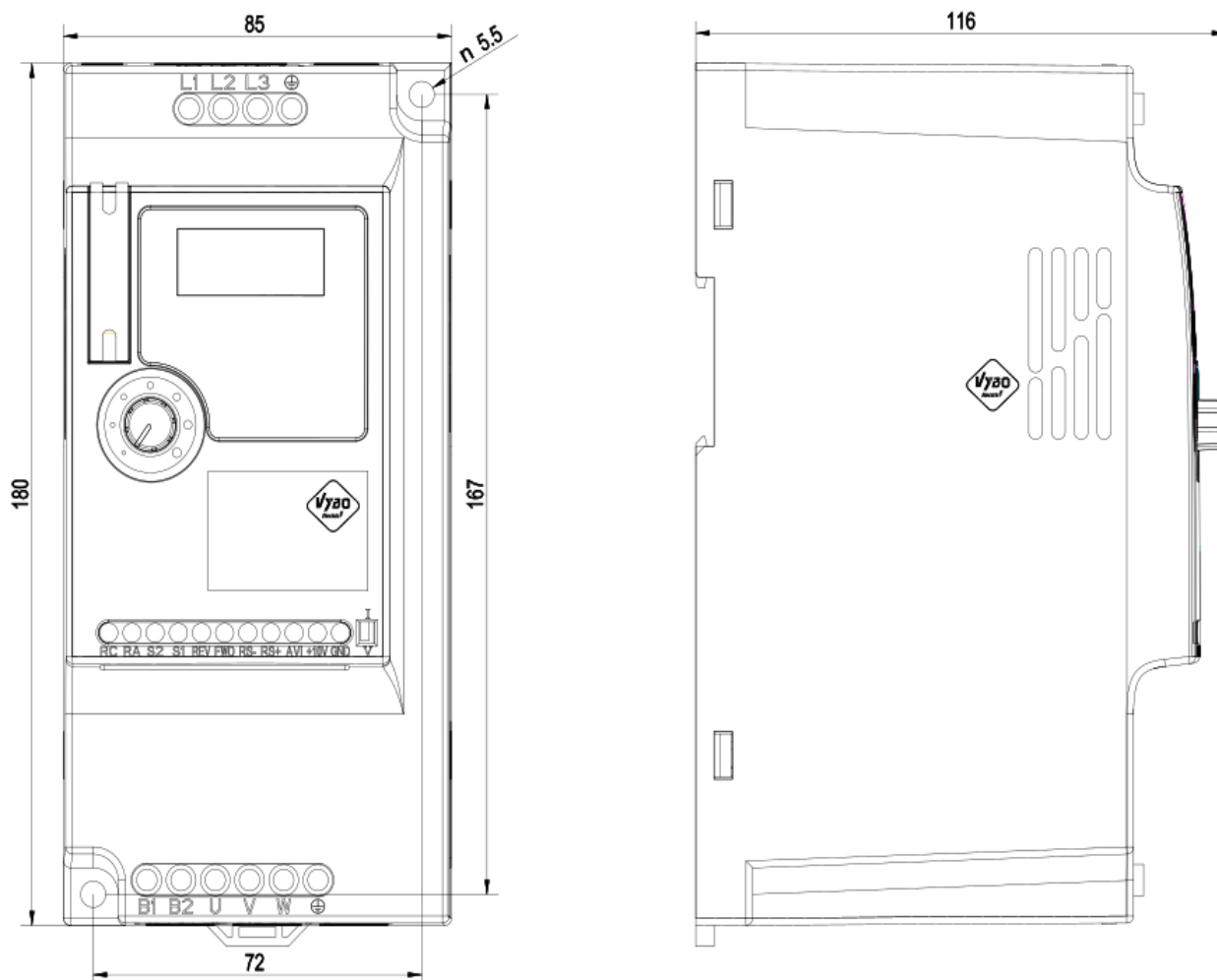
Rozmerový výkres A550 PLUS - 5,5kW 4T0055
