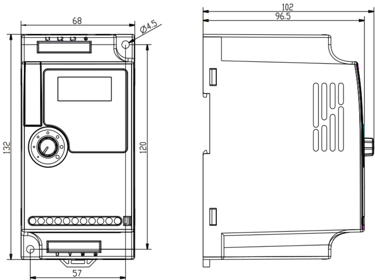
Rozmerový výkres A550 PLUS - 0,4kW 2S0004
