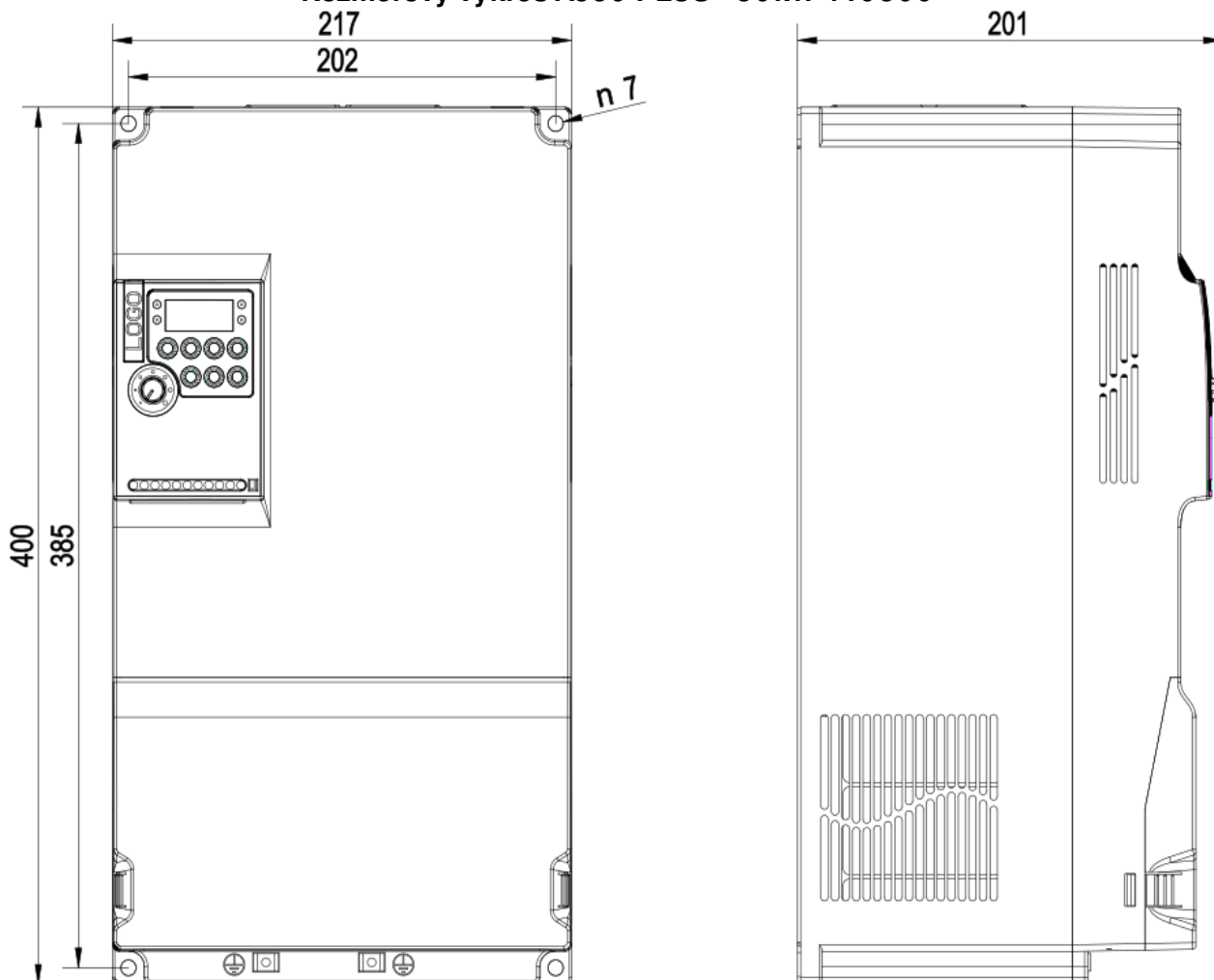
Rozmerový výkres A550 PLUS - 30kW 4T0300
