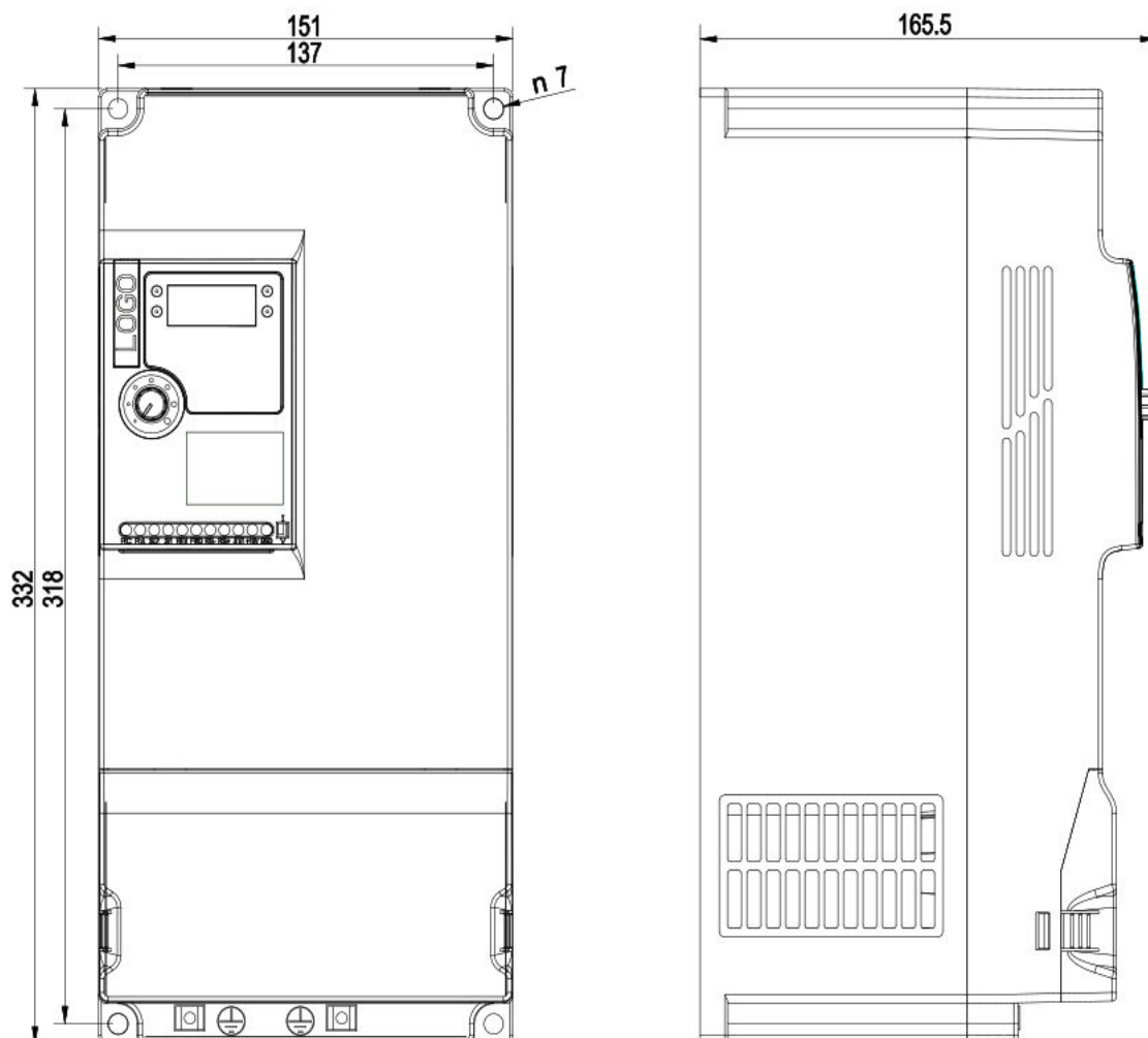
Rozmerový výkres A550 PLUS - 15kW 4T0150
