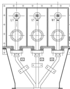
Typ D- terminál s úplne oddelenými fázami
