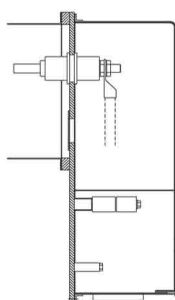
Typ C - terminál s oddelenými fázami
