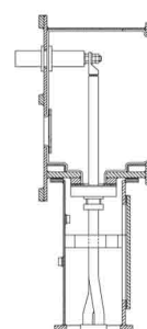
Typ D- terminál s úplne oddelenými fázami
