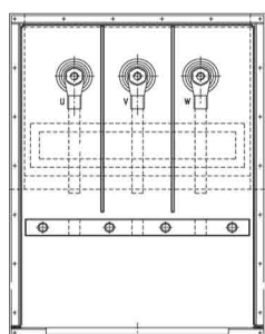
Typ C - terminál s oddelenými fázami
