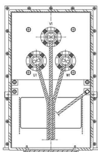
Typ A - veľký terminál
